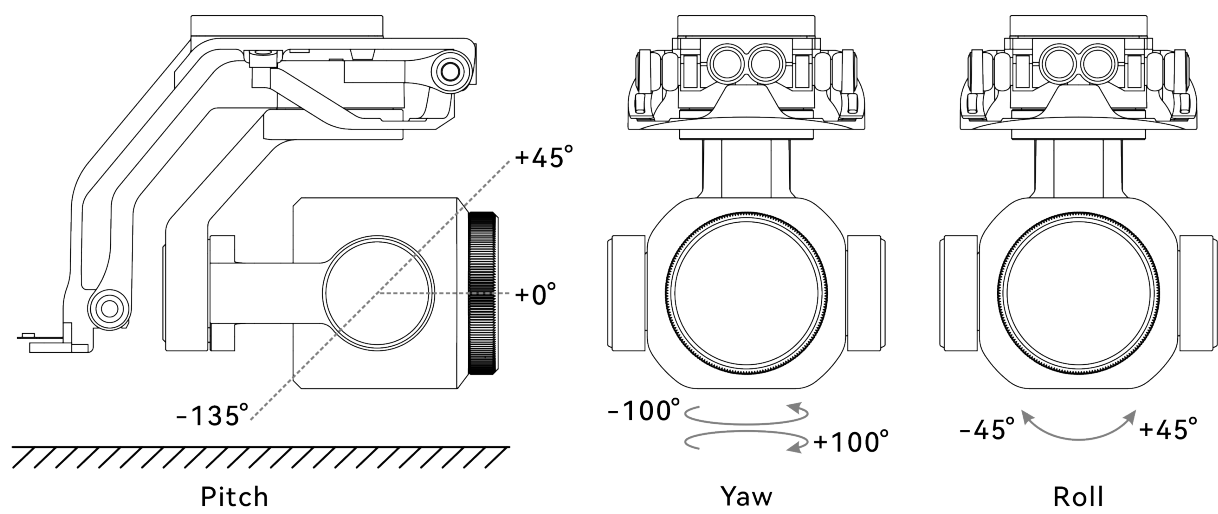
图 3-13 EVO II Pro V3 无人机云台机械转动范围
