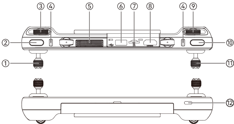
图 4-1 遥控器顶视图/底视图
