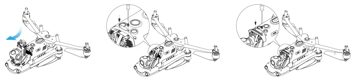
图 3-15 安装云台
