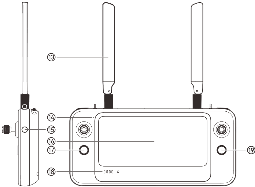
图 4-2 遥控器右视图/正视图
