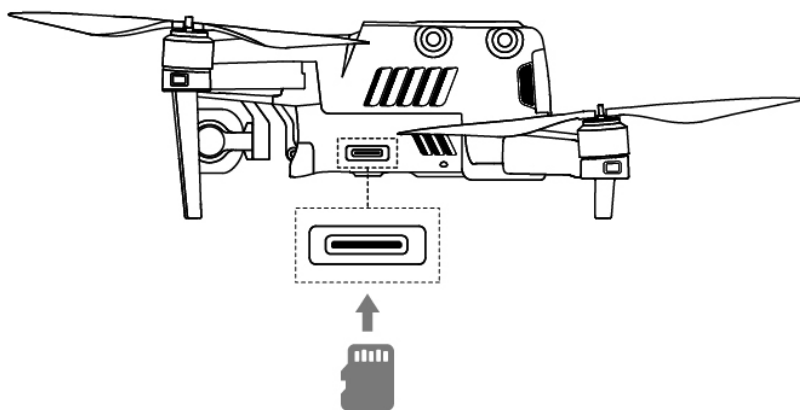
图 3-16 安装 microSD 卡
