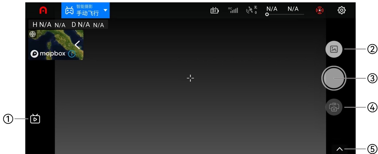
图 6-7 相机页面
