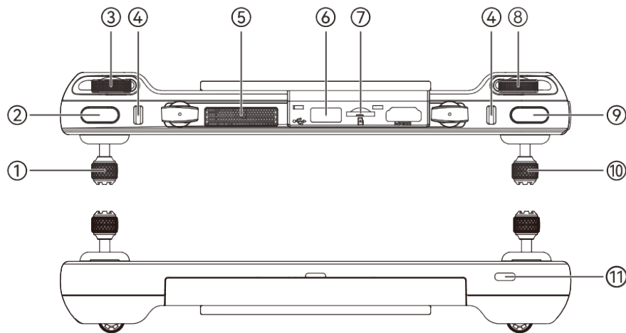
图 4-1 遥控器顶视图/底部图
