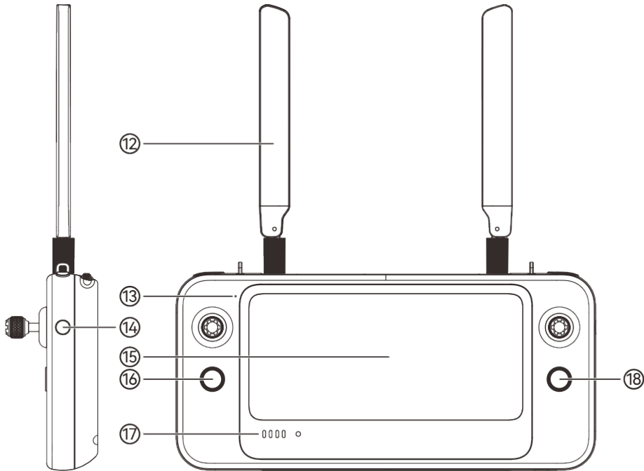
图 4-2 遥控器右侧视图/正视图
