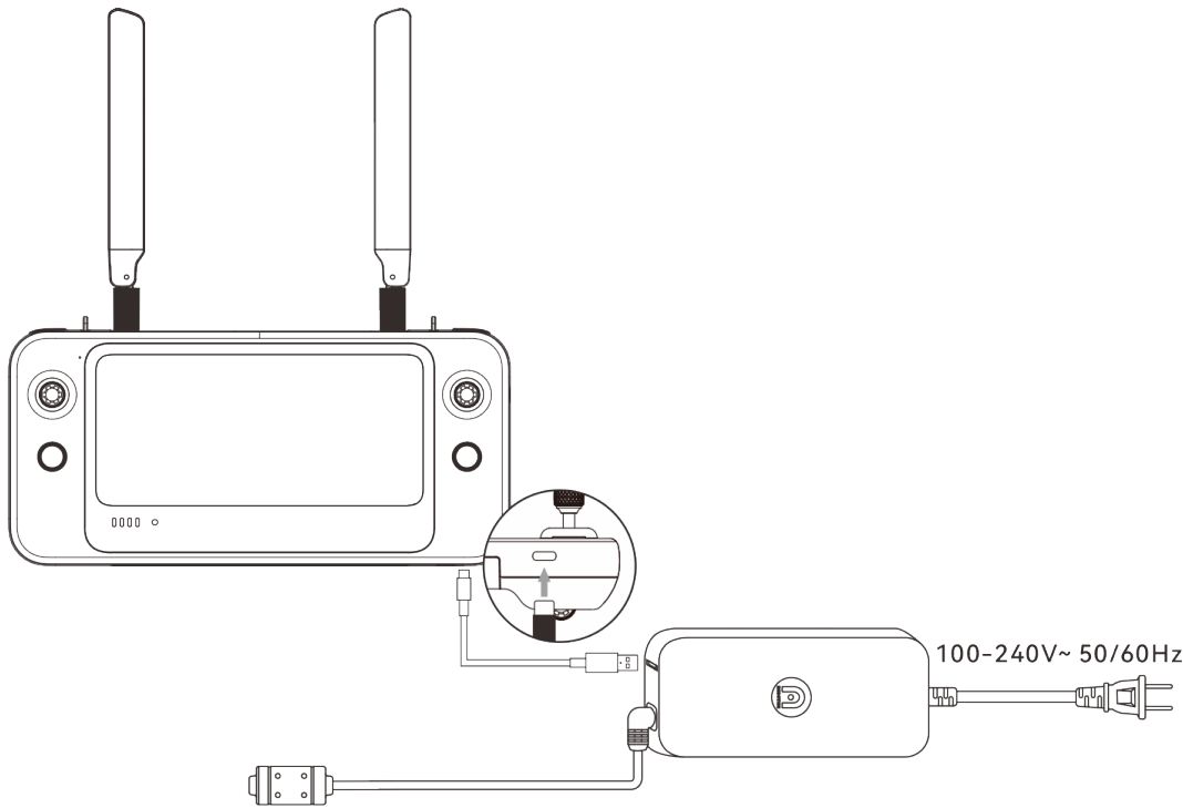
图 4-8 通过电池充电器给遥控器充电
