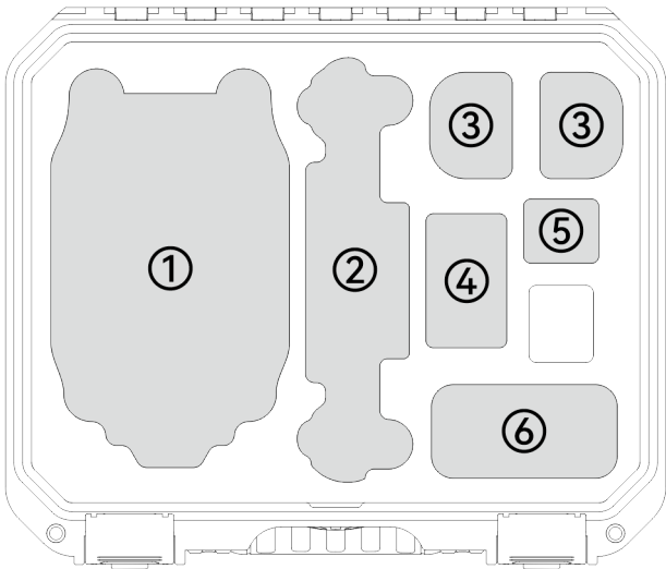
图 1-2 套装版装箱示意图
