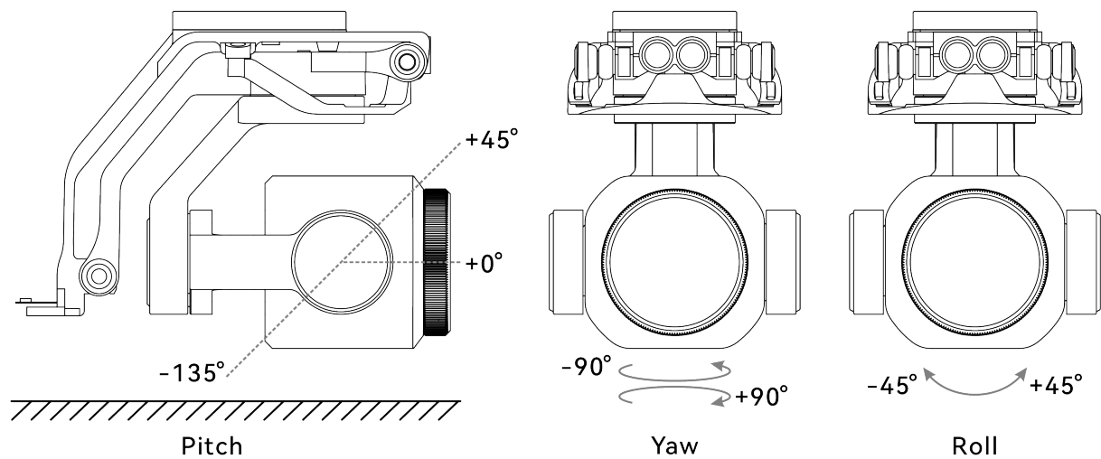
图 3-11 EVO Lite 6K 行业版的云台机械转动范围
