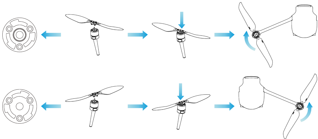
图 3-5 螺旋桨安装示意图
