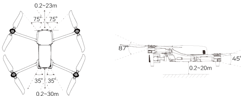
图 2-1 无人机视觉避障感知范围
