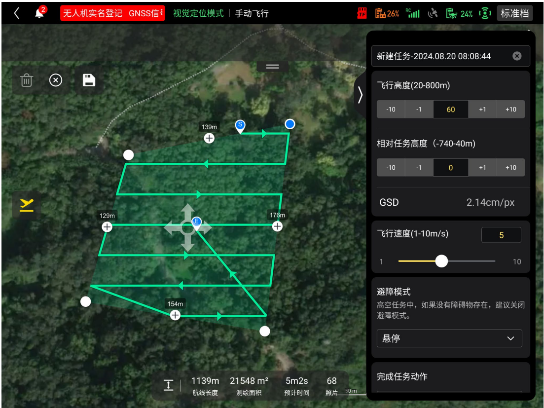
图 6-16 “多边形任务”页面（未起飞前）
