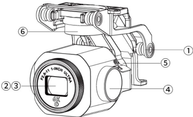
图 3-10 EVO Lite 6K 行业版的云台
